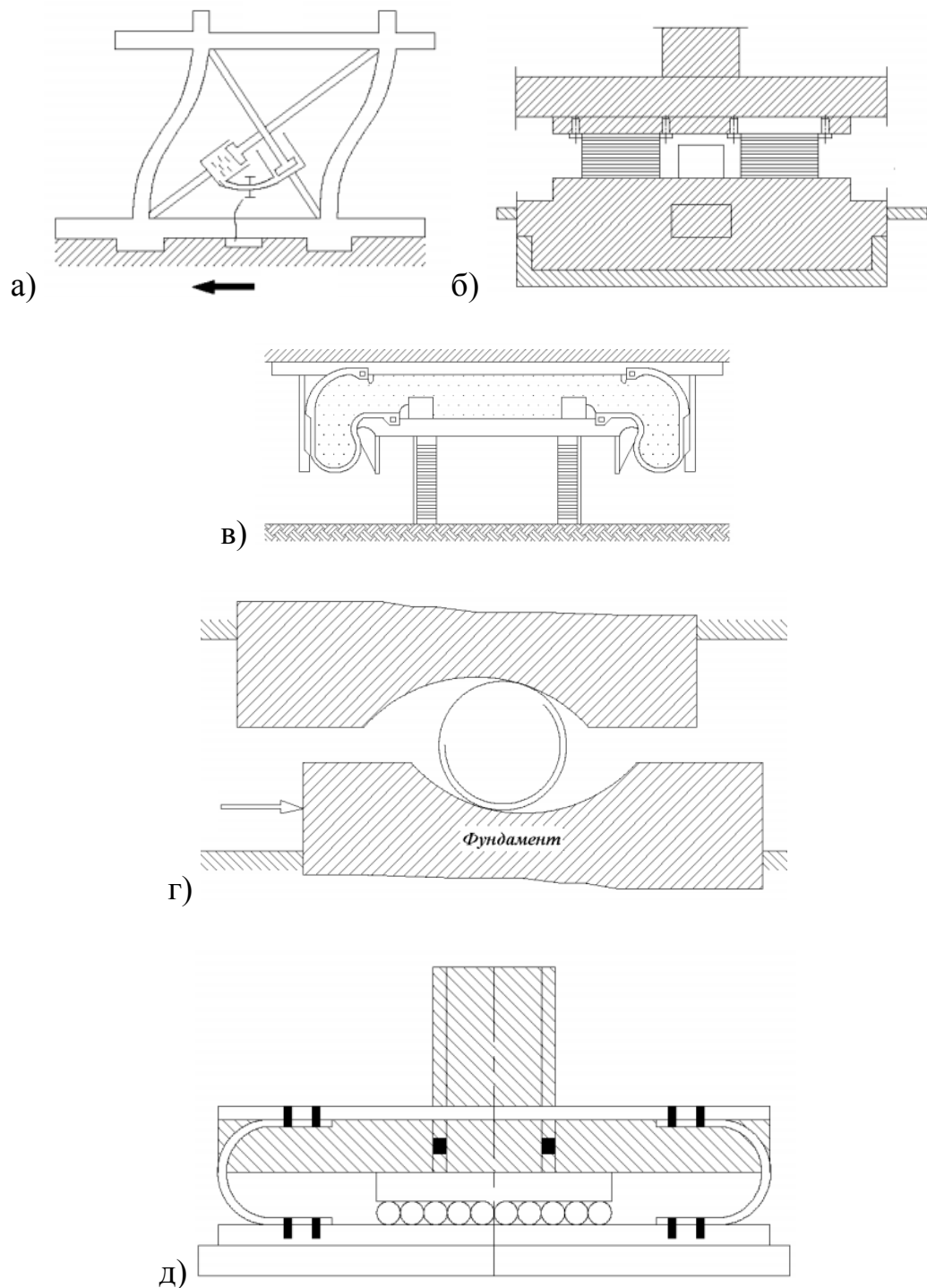
Рис. 2.10. Схеми активного сейсмосахисту місячного модуля: а - схема пристрою для зміни характеристик жорсткості та динамічних параметрів модуля; б - резинометалевий сейсмоізолятор; в - сейсмоізолятори з повітряною по душкою високого тиску; г-сейсмоізолятор із ковзними поясами з використанням ефекту тертя-ковзання
