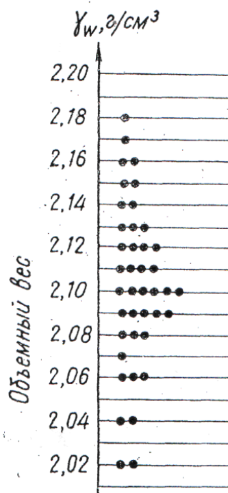
Рис. 1. Графік розсіювання значень об'ємної ваги ґрунту
