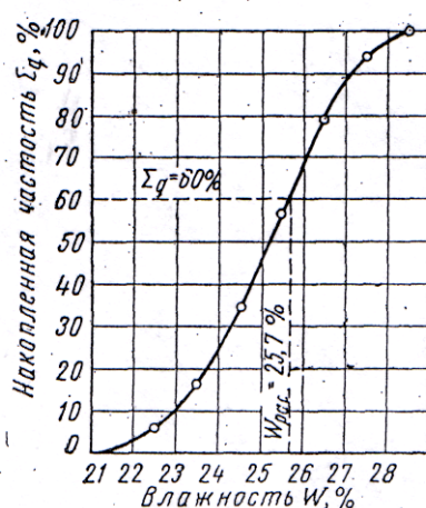
Рис. 2. Кумулятивная кривая значений влажности грунта
