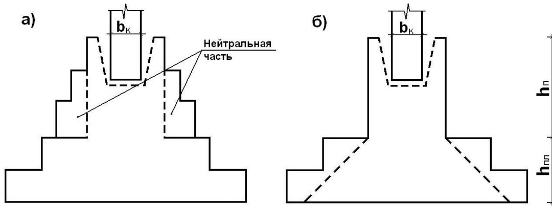
Рис. 3.2. Схема конструювання фундаменту з підвищеною стаканною частиною: а) масивний фундамент; б) фундамент з підколонником.
