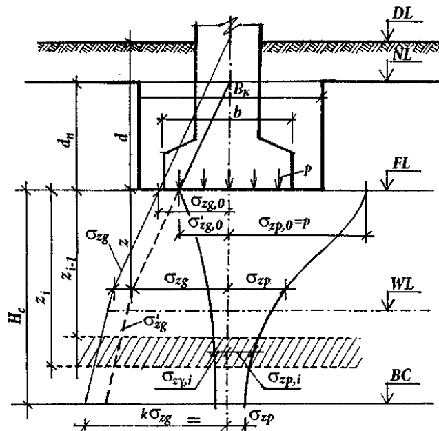
Рис. 3.1. Схема розрахунку осадок фундаменту методом пошарового підсумовування для схеми лінійно-деформованого півпростору DL - позначка планування підсіпкою (або зрізкою); NL - позначка поверхні природного рельєфу; FL - позначка підшви фундаменту; WL - позначка рівня підземних вод; BC - нижня межа стисливої товщі; d і d_n - глибина закладання фундаменту відповідно від рівня планування і поверхні природного рельєфу; H_c - глибина стисливої товщі; b - ширина фундаменту; B_k - ширина котловану; p - середній тиск під підшовою фундаменту; \sigma_{zg} і \sigma_{zg,0} - вертикальне напруження від власної ваги ґрунту на глибині z від підшви фундаменту і на рівні підшви з врахуванням планування поверхні ґрунтової основи підсіпкою (або зрізкою); \sigma_{zp} і \sigma_{zp,0} -
